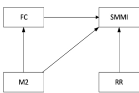
图 3 有向无环图
